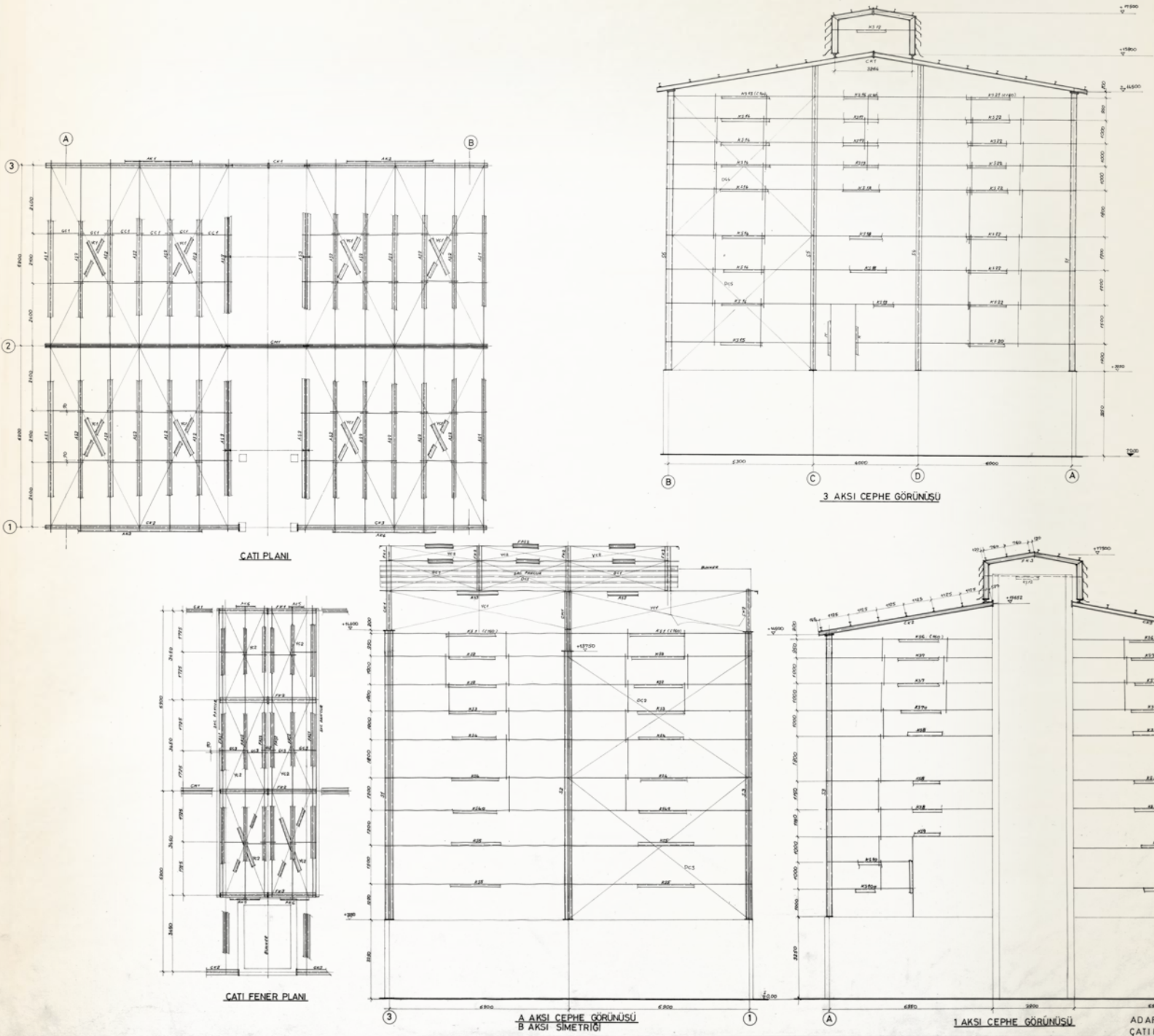
1950'lerin başı Adapazarı Nişkoz Fabrikası inşaat planı
